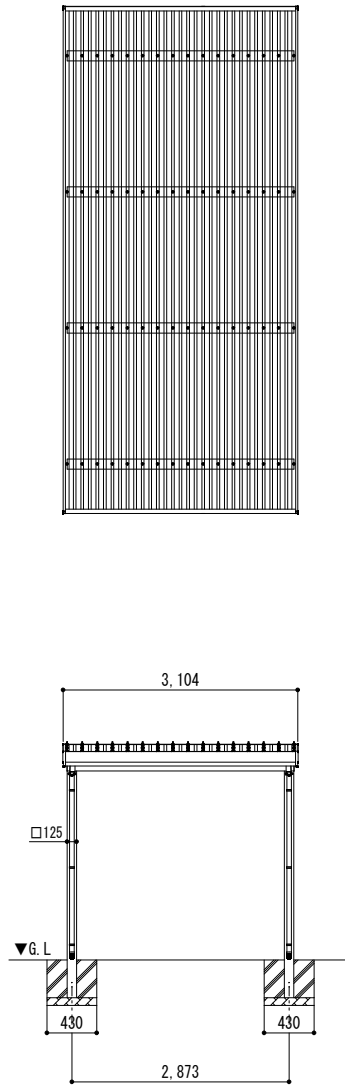
■ 立面図
