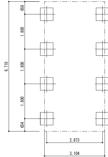
■ 基礎配置図
